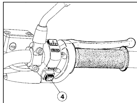
FIG. 11 1. Commutateur de démarrage 2. Levier du starter 3. Commutateur droit 4. Bouton de démarrage moteur
